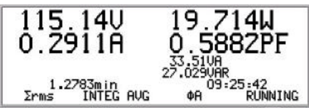
Figure 28. Basics àRMS INTEGR AVG fA display
